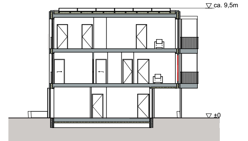
Doorsnede A-A
